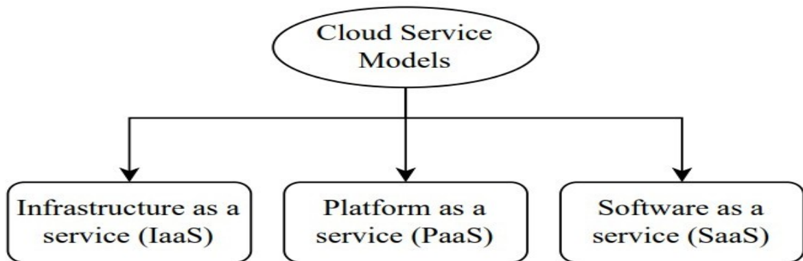
Fig.2:CloudServiceModels
